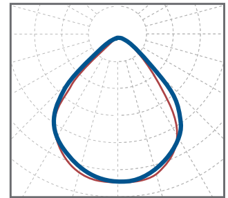
Г90 КСС 90°
