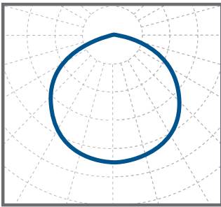
Д КСС 120°
