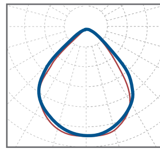
Г90 КСС 90°
