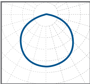
Д КСС 120°
