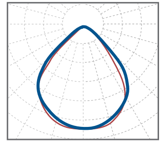
Г90 КСС 90°
