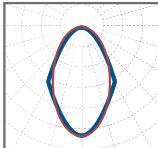
К60 КСС 60°
