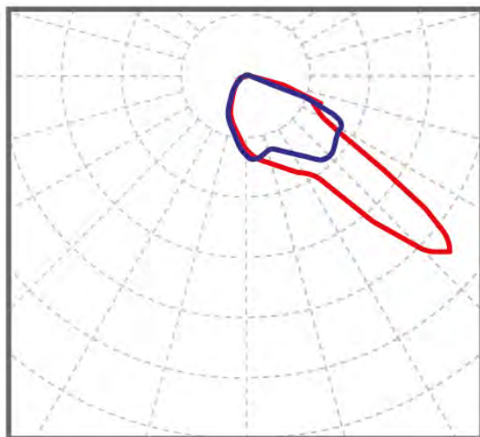
асимметричная КСС 90°x20°
