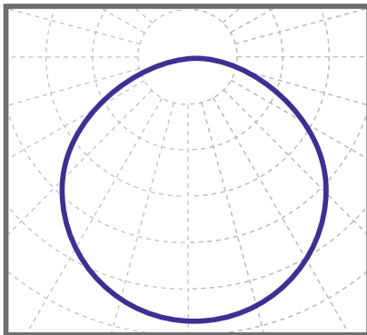
косинусная КСС 115°
