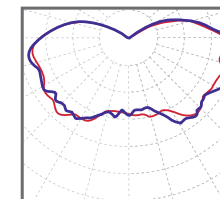
широкая КСС 180°
