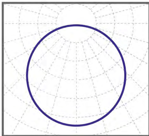
косинусная КСС 120°
