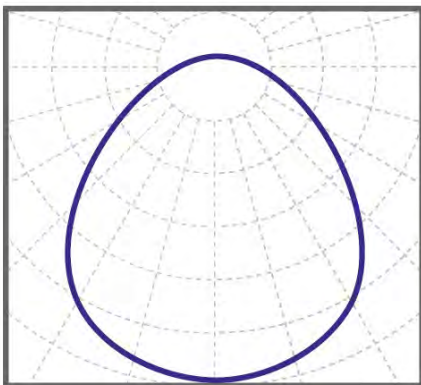
Diora NPO Mini Prism
