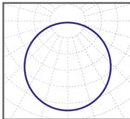
Diora NPO Mini Opal
