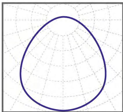
косинусная КСС 90°
