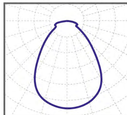
косинусная КСС 80°
