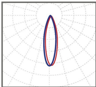
концентрированная 30°
