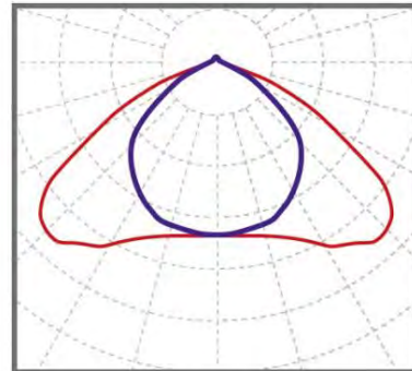
широкая осевая 125°x105°
