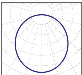
косинусная KCC 110°
