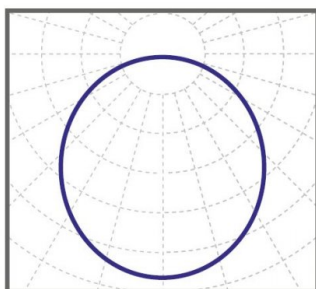
косинусная КСС 110°
