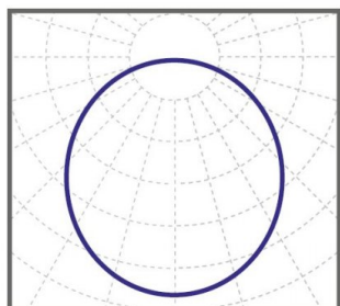
косинусная КСС 110°
