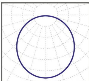
косинусная КСС 110°
