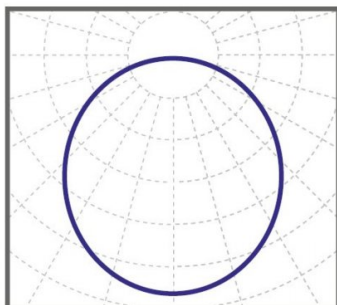
косинусная КСС 110°
