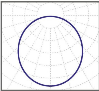
косинусная КСС 110°
