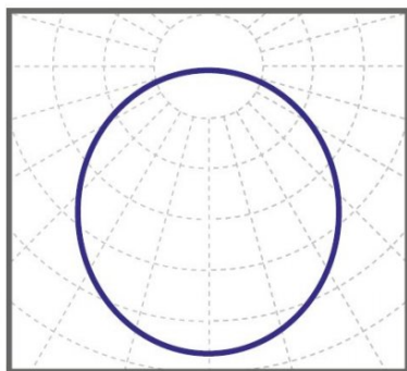
косинусная КСС 110°
