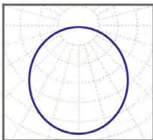
косинусная КСС 110°
