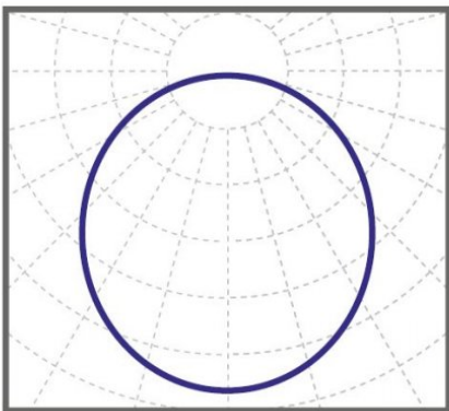
косинусная КСС 110°
